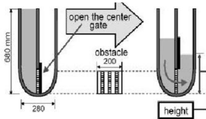
Fig: U-Box
