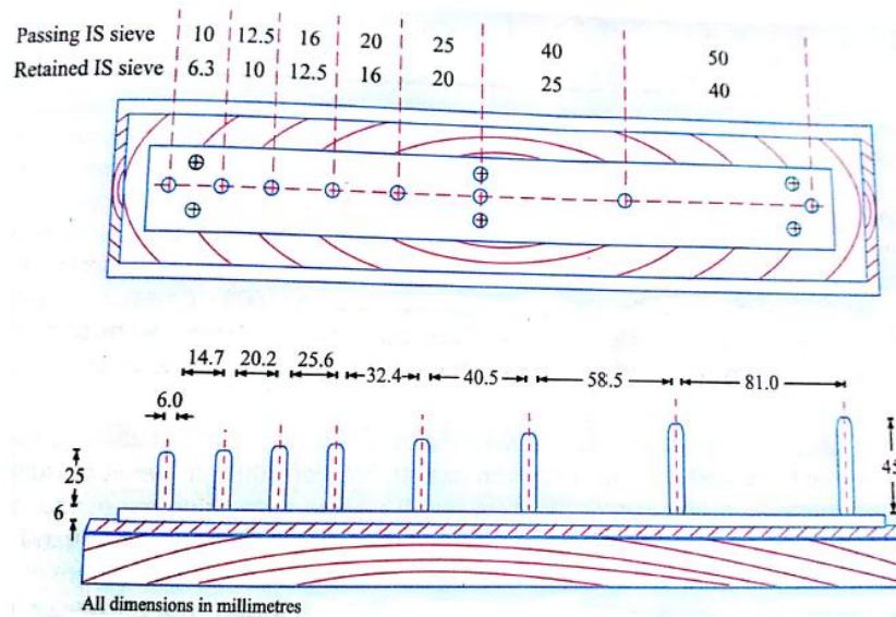
Fig. 3.10. Length Gauge.
