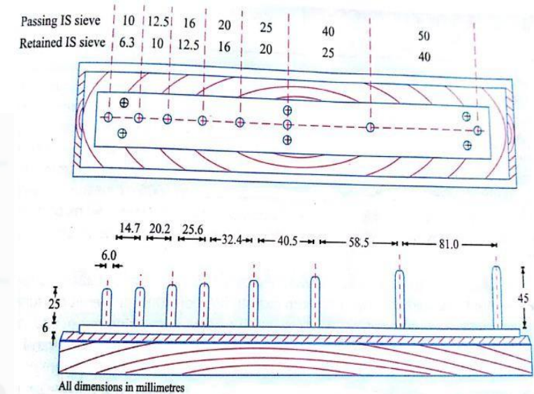
Fig. 3.10. Length Gauge.
